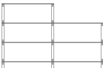
Comp. 10 - 195 x 40 h. 126 cm
